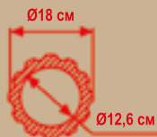
90018-1 (30 x 36 x 36 cm)
